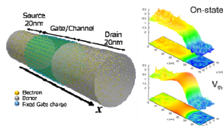
ナノスケールトランジスタの動作シミュレーション
