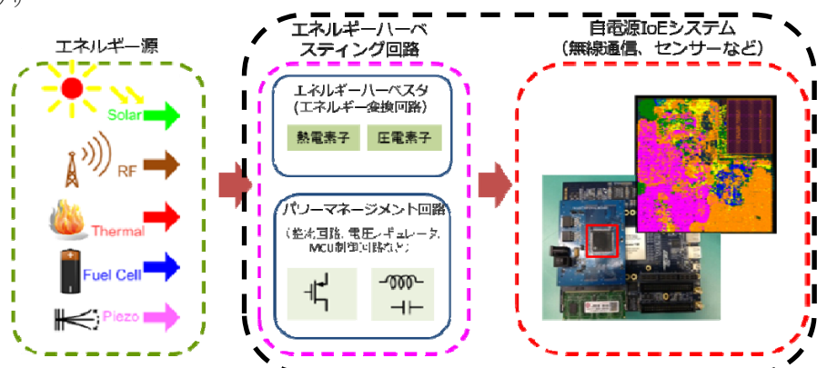
発電・センシング一体化システム
