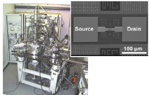
シングルイオン注入装置と単ドーパントデバイス
