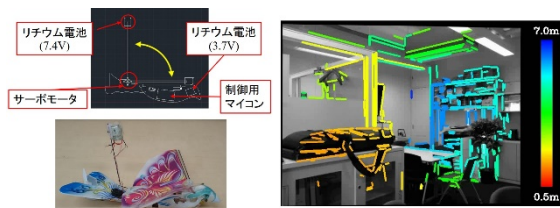
羽ばたき型飛行ロボットとロボットビジョン
