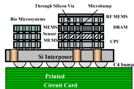
3次元積層集積回路の概念図
