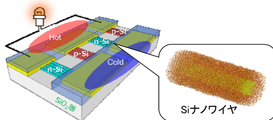
オン・シリコン熱発電デバイス
