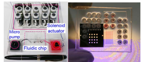
4x4マイクロチャンパーを持つマイクロ化学反応システム
